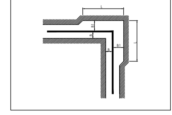
Udformning af ekspansionszoner, nedlægningsmetode 1 og 4 i.h.t. Isoplus's katalog.
